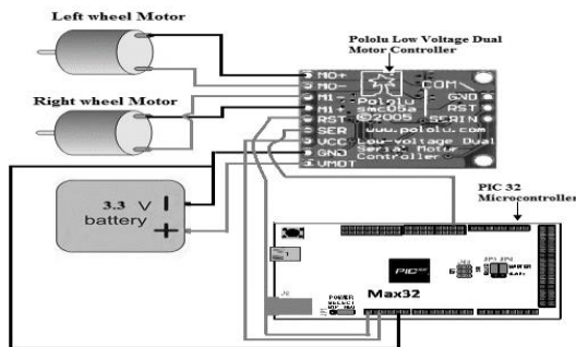
Fig. 5 – Motor Controller Wiring
